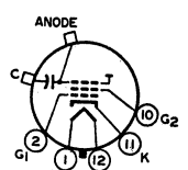
12N ANODE = G_3 + CL
